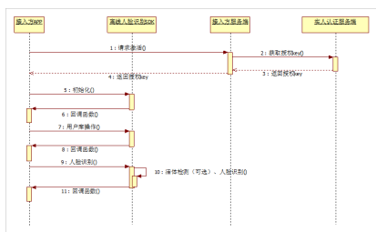
图 2-1: 离线人脸识别SDK接入时序图
