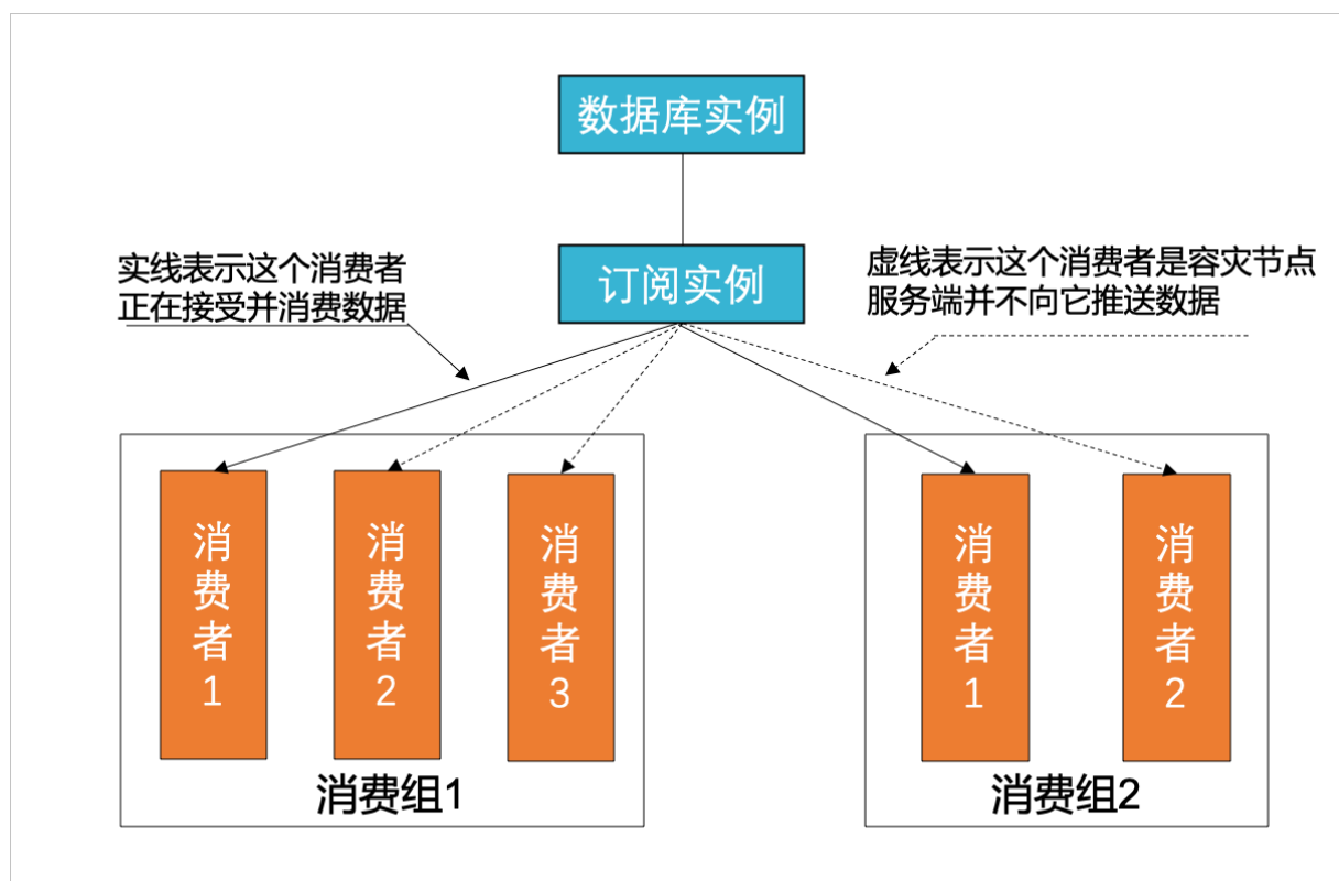
图 3-1: 消费组架构
