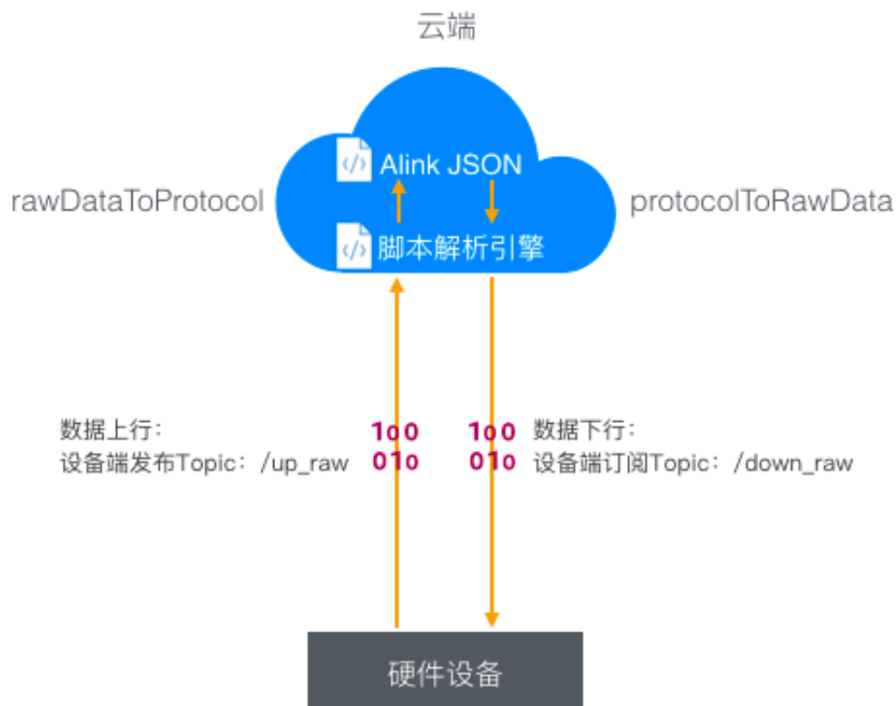
设备上报透传格式的属性或事件（上行数据）全流程图：
