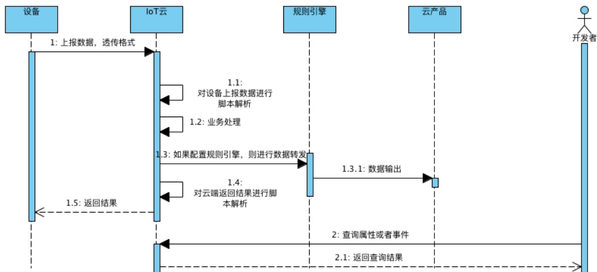
调用设备服务或设置属性（下行数据）全流程图：
