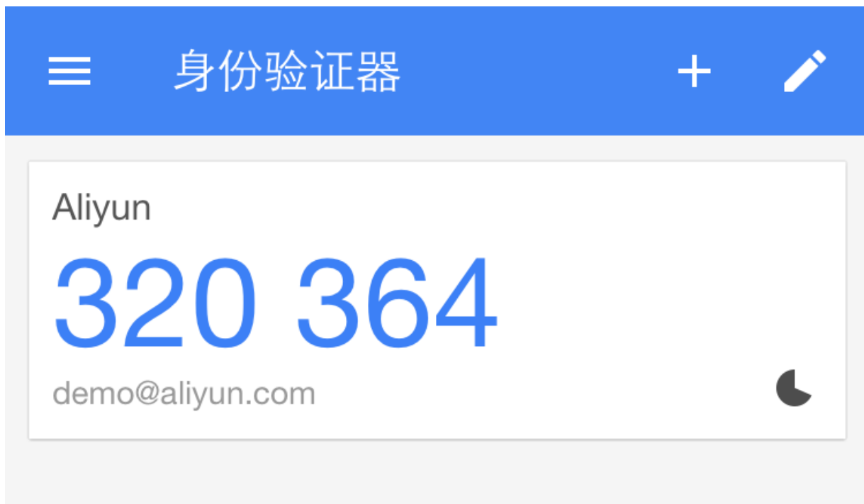
图 8-3: 身份验证
