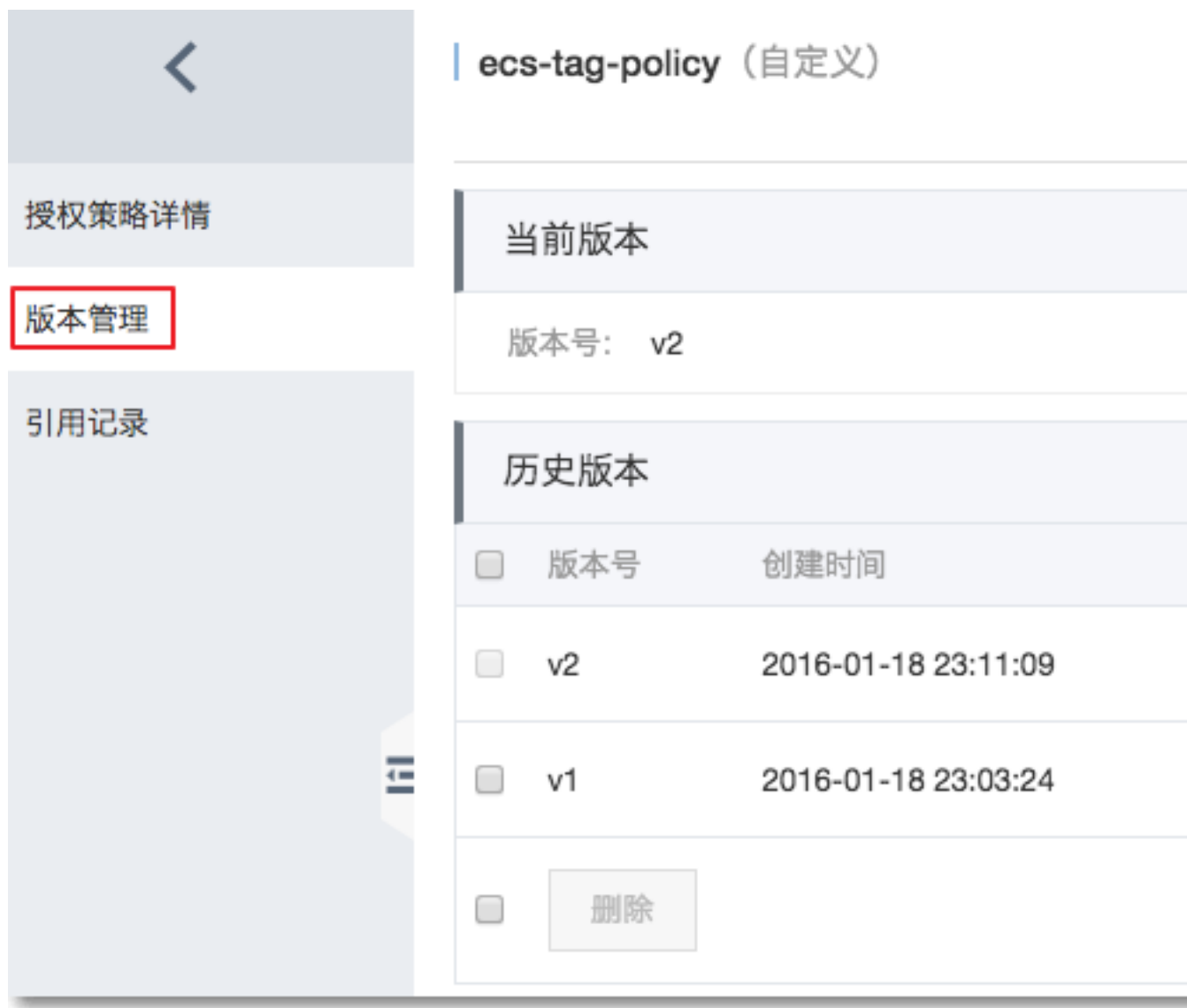
图 3-3: 版本管理
