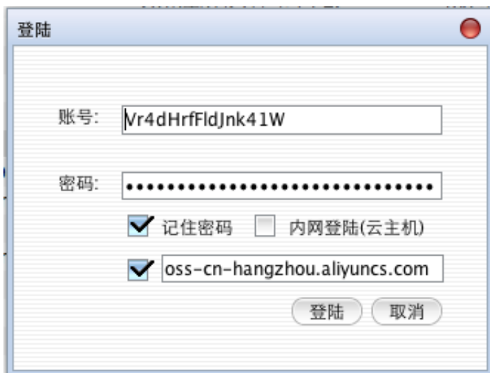
图 3-4: 登录
