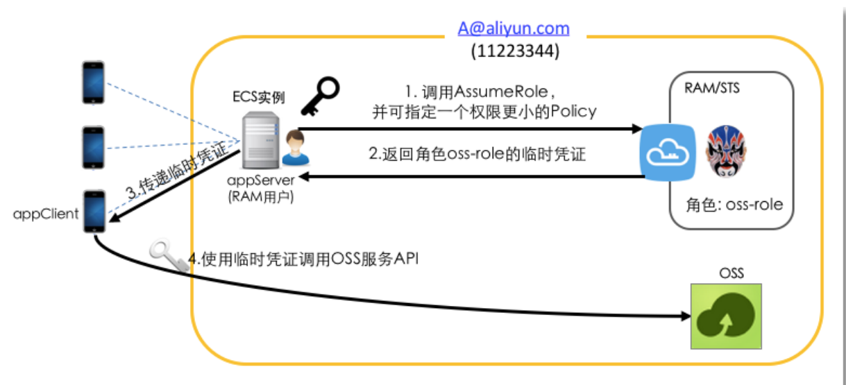
图 6-2: 操作流程
