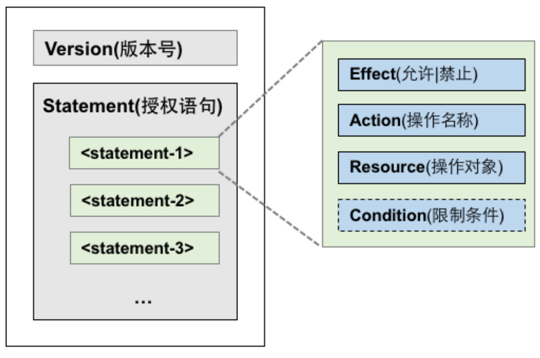
图 4-1: Policy结构
