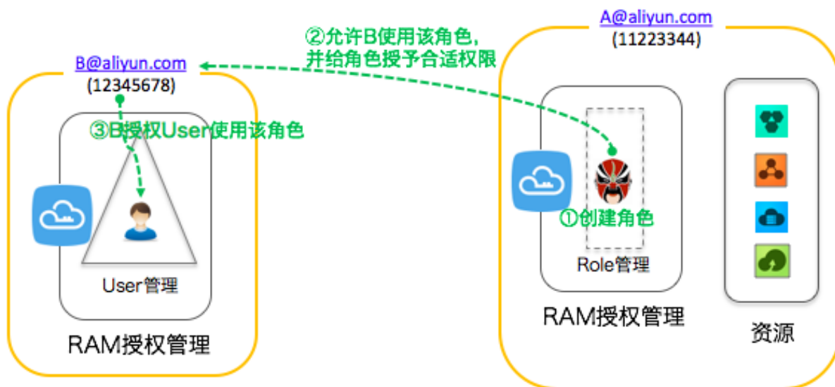
图 6-3: 跨账号授权
