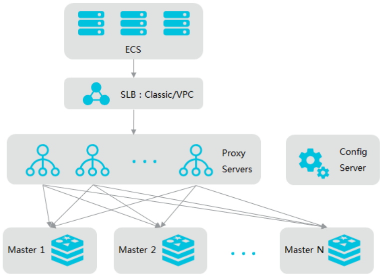
集群版代理模式组件说明
