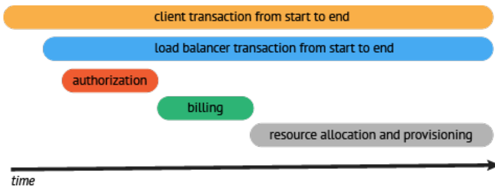
图 2-2: 包含时间轴的链路图
