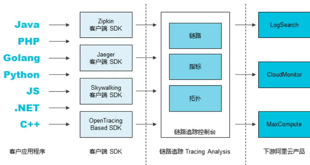
图 1-1: 链路追踪产品架构
