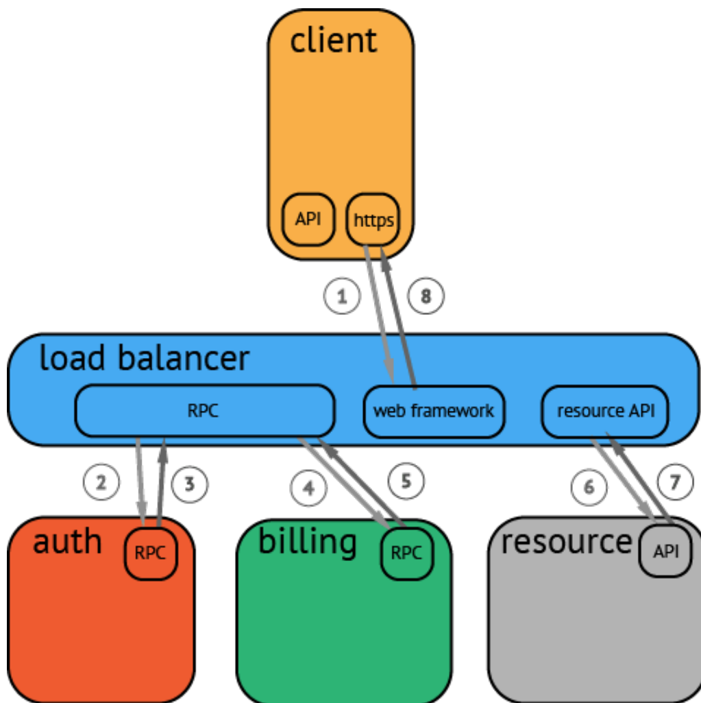
图 2-1: 分布式调用示例
