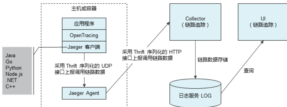
图 2-4: 通过 Agent 上报数据
